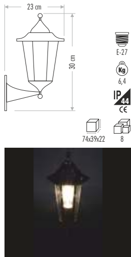
CT-7035 ABS PLASTİK 70,00 ₺
