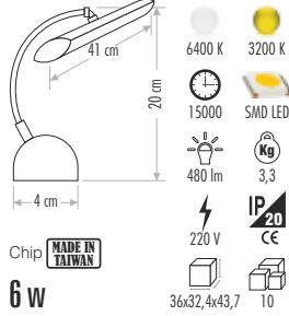
CT-5246 KUĞU LEDLİ APLİK 135,00 ₺
