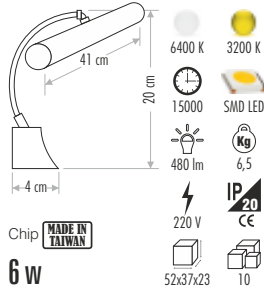
CT-5247 PELİKAN LEDLİ APLİK 130,00 ₺
