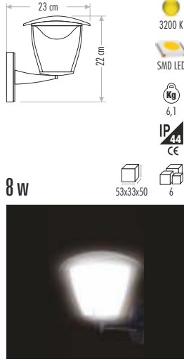
CT-7070 AKAY LED APLİK 195,00 ₺
